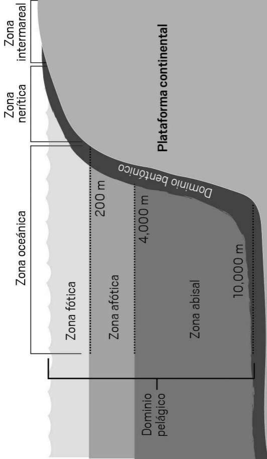
Figura 5: Descripción gráfica de la ubicación de las zonas fótica/afótica como distribución de la luz en el océano.
