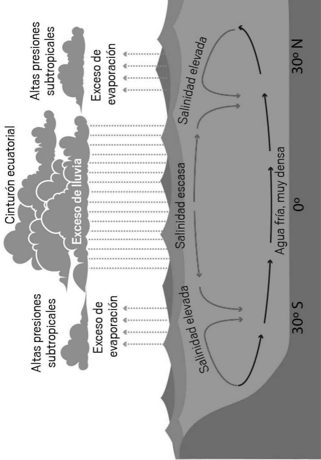
Figura 28: Salinidad en el agua de mar.
