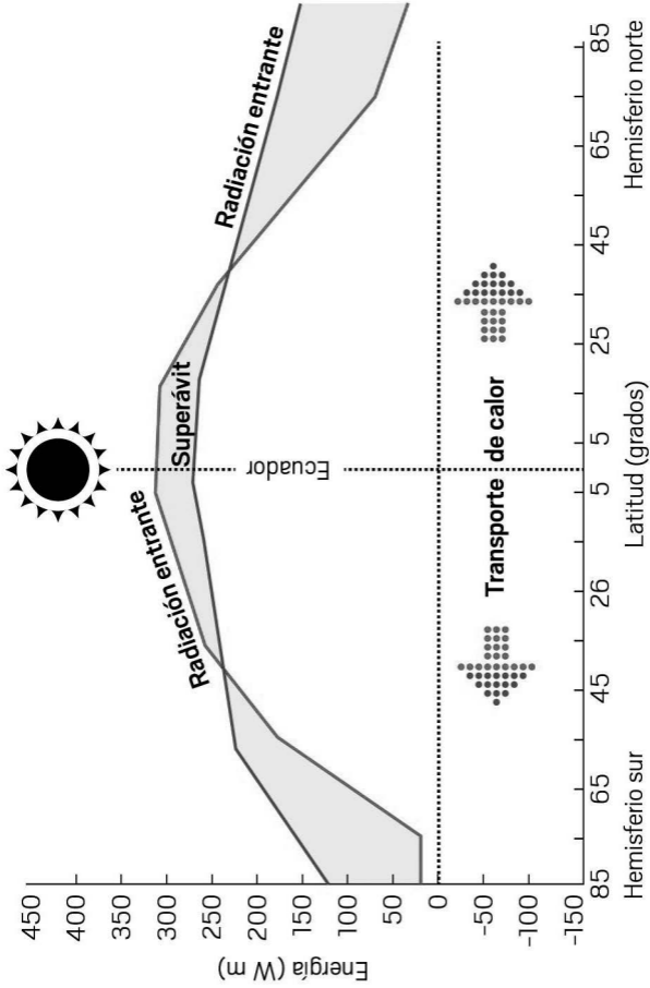
Figura 7: Balance radiativo anual. La mayor incidencia de luz solar en el ecuador genera una diferencia en la distribución de calor y energía sobre el planeta.
