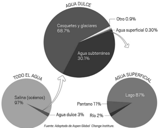
Figura 21: Distribución del agua en el planeta.
