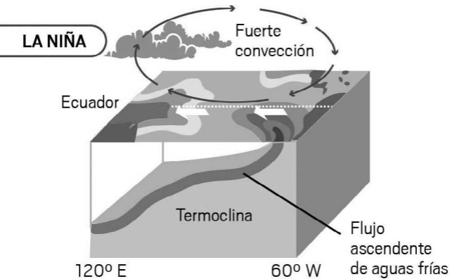
Figura 8: Diagramas de los cambios oceanográficos en el océano Pacífico durante los periodos de El Niño y La Niña.
