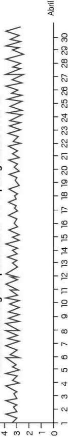
Figura 20: Variación del ciclo de mareas en la costa chilena.
