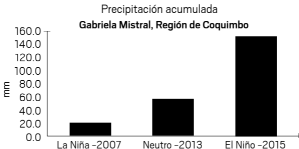
Figura 9-b: Precipitación acumulada en Gabriela Mistral en años influenciados por eventos La Niña, Neutro y El Niño (fuente: CEAZA-Met).
