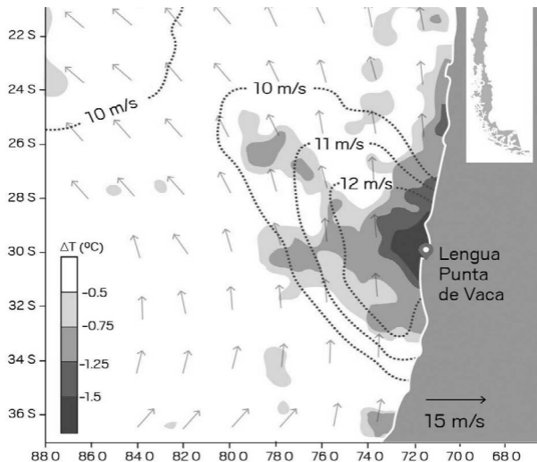
Figura 11: Evento de surgencia frente a la costa de la Región de Coquimbo.
