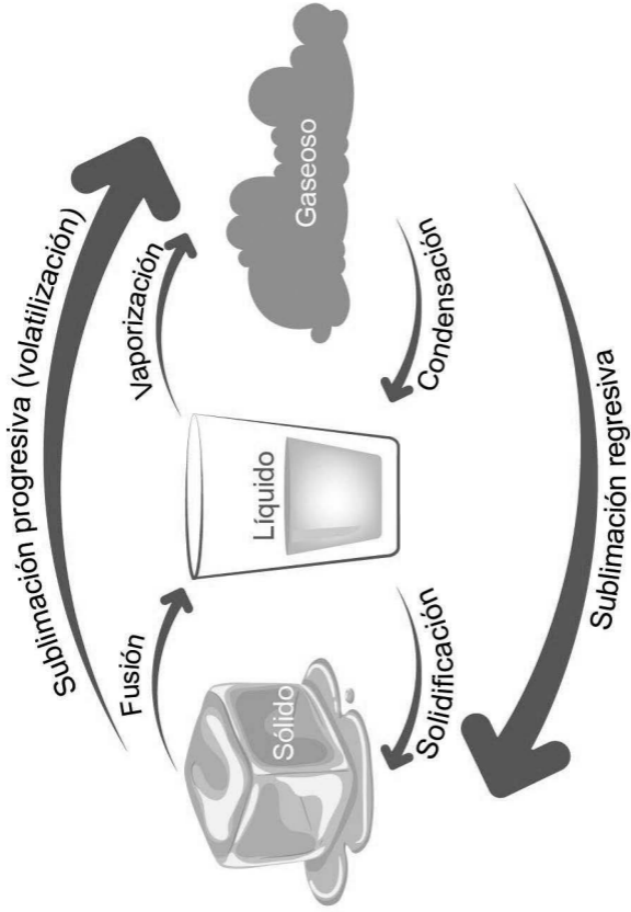
Figura 22: Cambios en las propiedades del agua.
