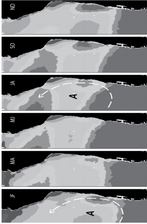
Figura 12: Climatología bimensual de la velocidad del viento ( m/s^{-1} ) en el océano.
