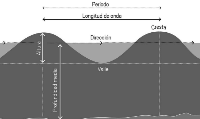
Figura 17: Características de las olas.
